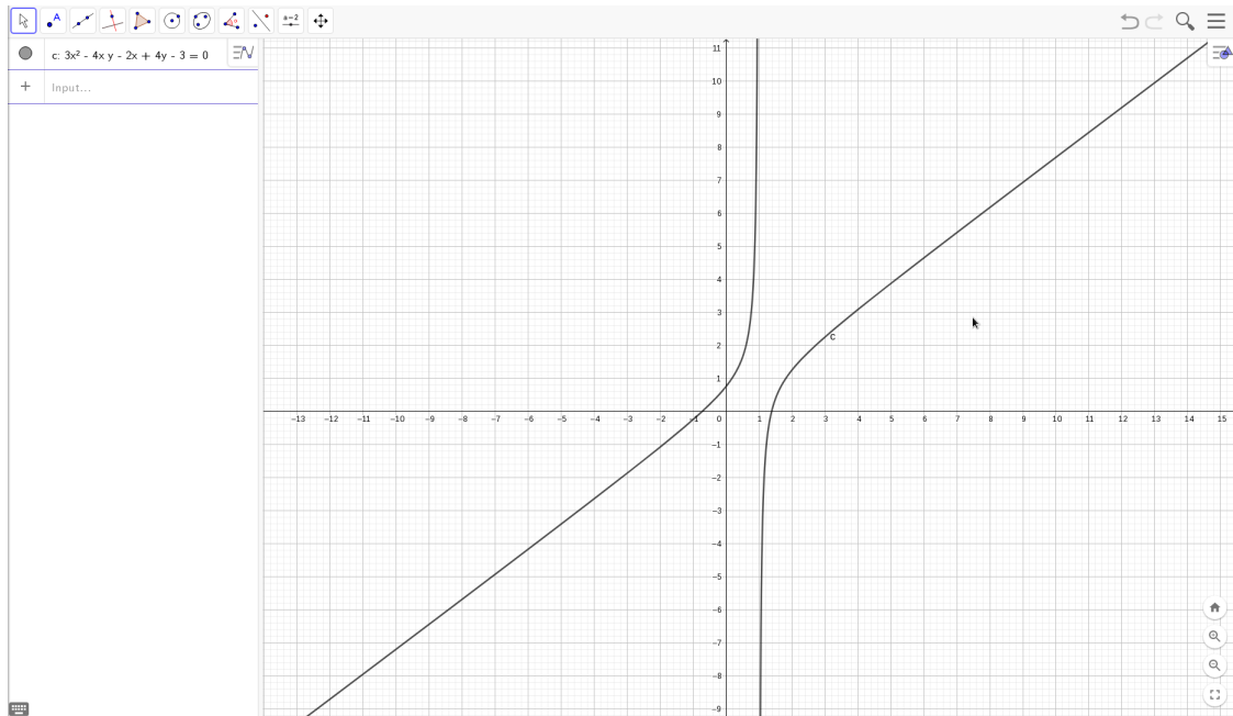
Figura 6.2: Hiperbola 3x^2 - 4xy - 2x + 4y - 3 = 0
